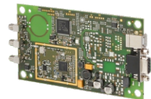
UHF Mid Range Reader Module ID ISC.MRMU102
